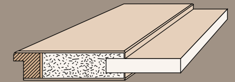
Rahmentür: echte Rahmenbauweise, Füllung eingeschoben
