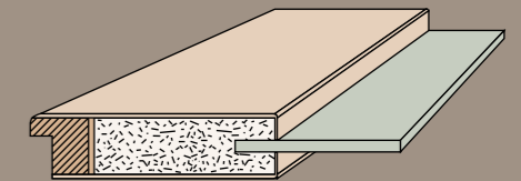
Tür mit Lichtausschnitt: Glas eingeschoben
